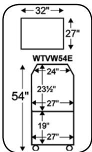
WTVW Cart Dimensions
