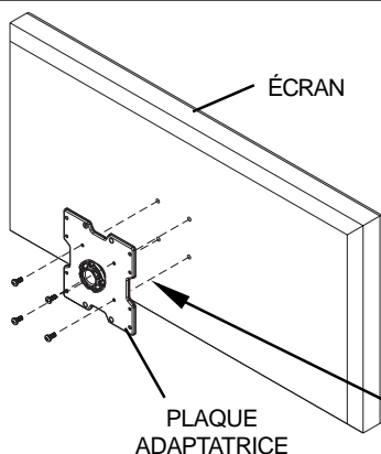
VESA® 100 x 100
