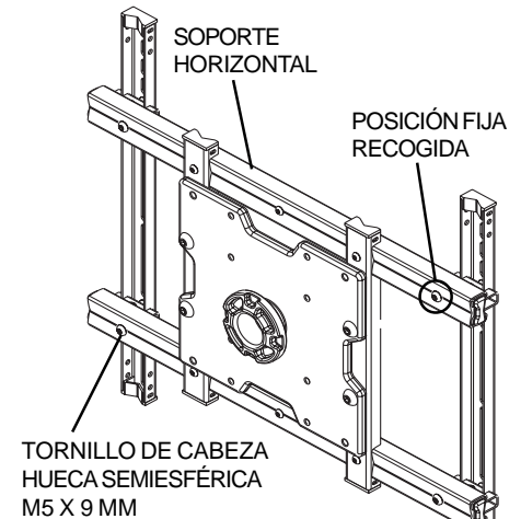
POSICIÓN RECOGIDA
