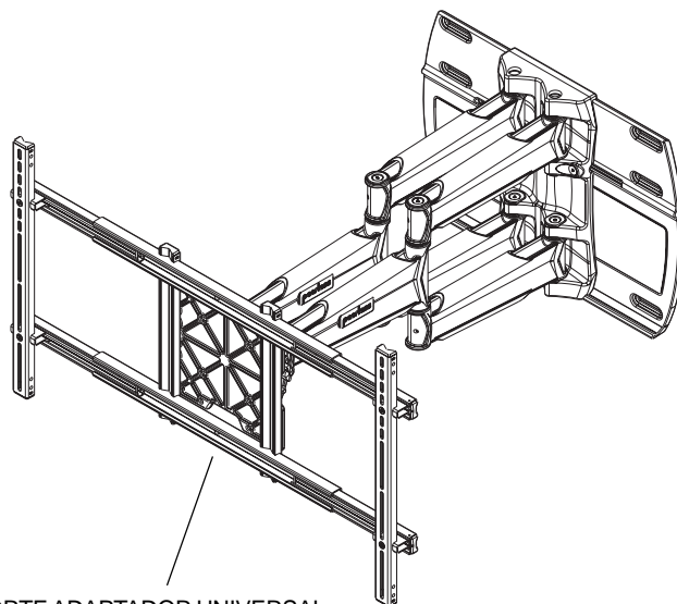
EL SOPORTE ADAPTADOR UNIVERSAL SE INCLUYE CON LOS MODELOS RTFPA63U, RTFPA63US, SA760PU, SA760PU-S
