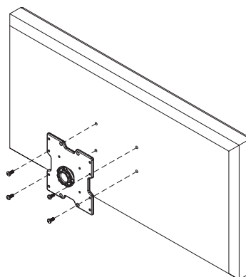
VESA® 200 x 100
