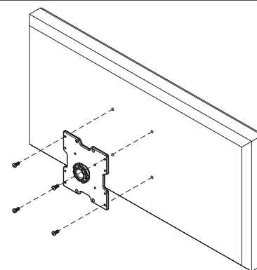
VESA® 200 x 200
