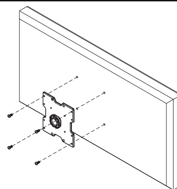
VESA® 200 x 200
